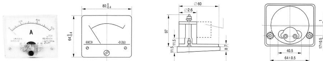
69L9、69C9、69L13 型电表
