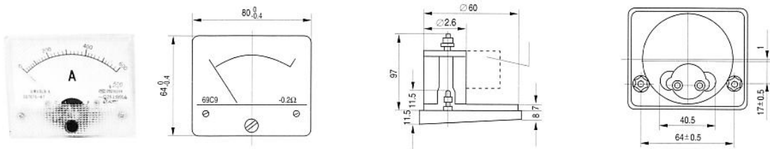
69L9、69C9、69L13 型电表
